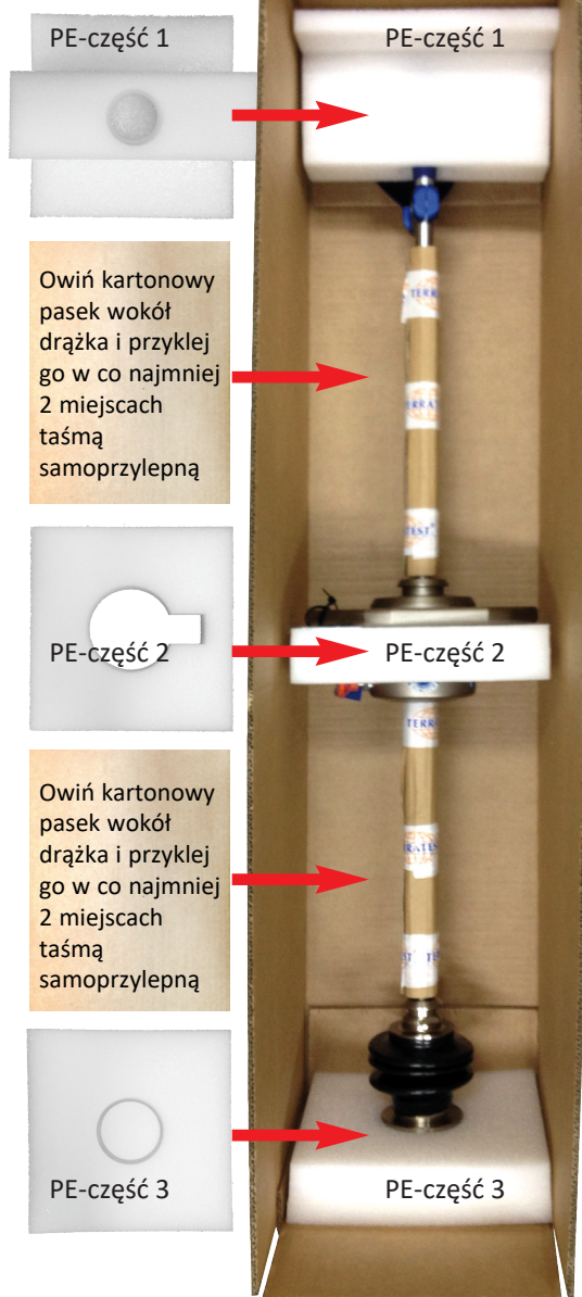
Rysunek 2: Urządzenie obciążeniowe
